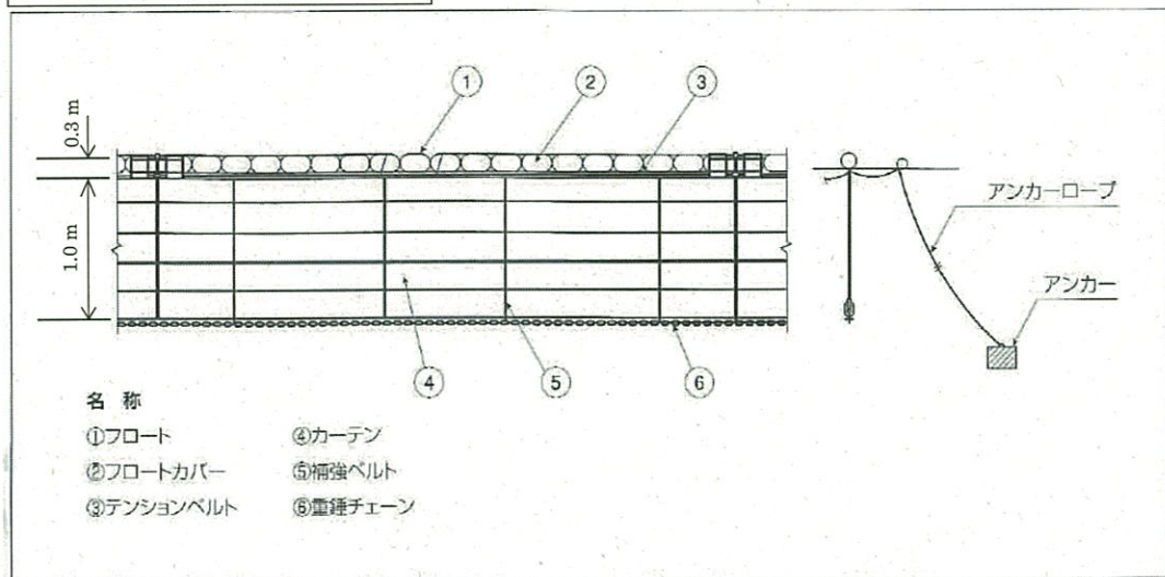
シルトフェンス 概略構造図
